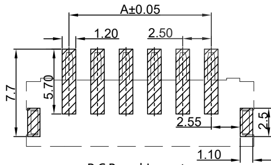
P.C.Board Layout
