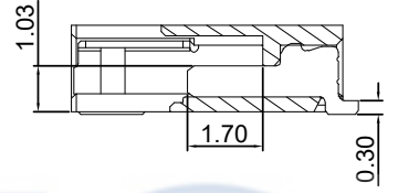
SECTION:A-A SCALE 1:1
