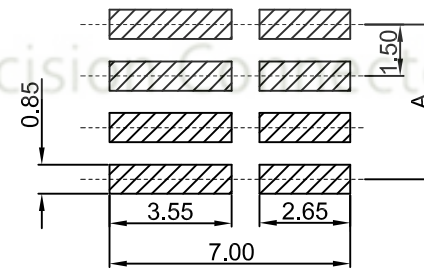
P.C.Board Layout
